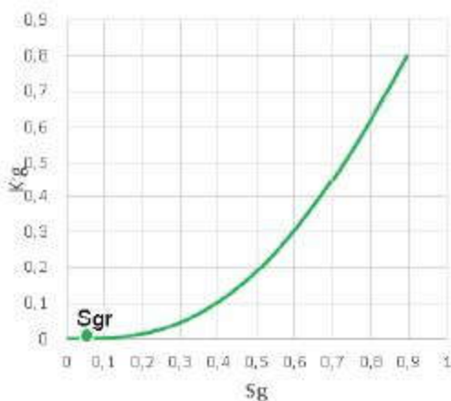
Рис.1. Типичные фазовые проницаемости воды и газа в гидрофильной пористой среде.
