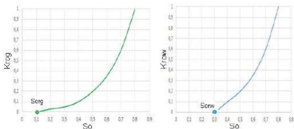
Рис.3. Типовые фазовые проницаемости нефти при двухфазной фильтрации с газом (слева), водой (справа).
